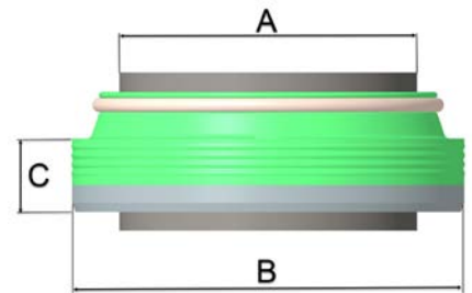
Design "A" - senza flangia Design "A" - w/o flange
