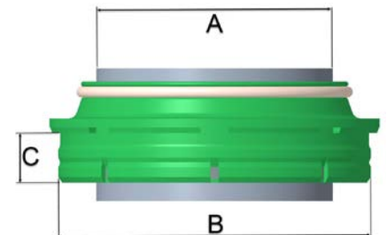
Design "B" - con flangia Design "B" - with flange
