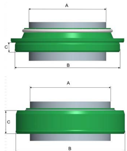
Design "C" - guarnizione e raschiatore in 2 parti Design "C" - seal and dust scraper in 2 parts
